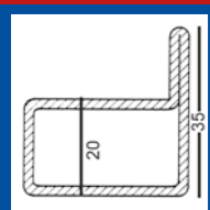
Profil RP 144
