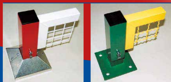
Höhenverstellbarer Fuß mit und ohne Abdeckung
